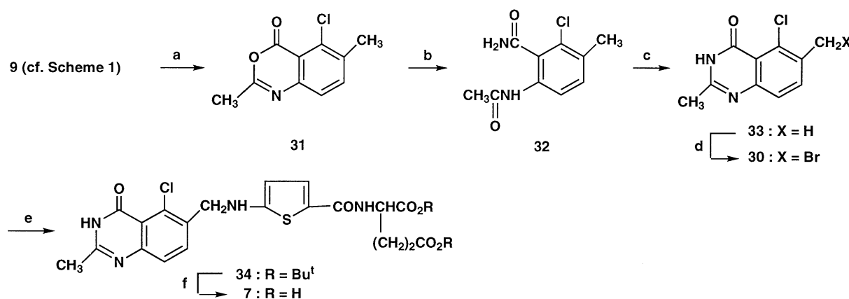
Scheme 3. Reagents: (a) \text{Ac}_2\text{O} , reflux; (b) \text{NH}_3 , -33^\circ\text{C} ; (c) 1 N NaOH, reflux; (d) NBS/ \text{Bz}_2\text{O}_2 , \text{CHCl}_3 (e) 28 , \text{NaHCO}_3 , DMF; (1) 1:3 TFA– \text{CH}_2\text{Cl}_2 , 5^\circ\text{C} .
